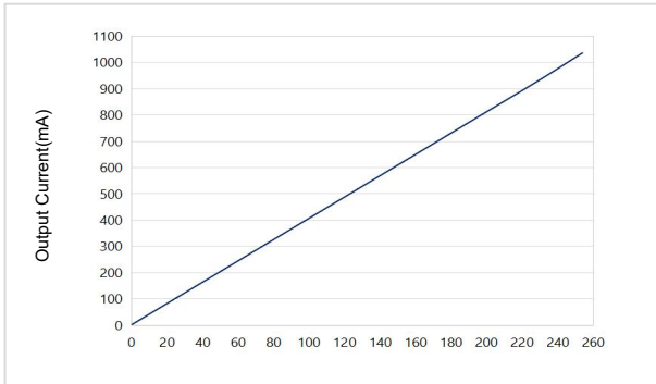
linear dimming
